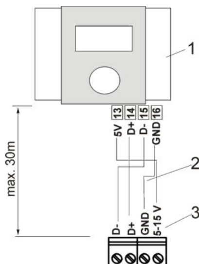
4-žilové zapojení pokojového panelu ecoSTER BN: 1 – ecoSTER BN, 2 – kabeláž, 3 – svorkovnice regulátoru BENEKOV EM 250
