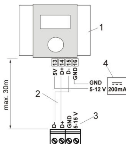
2-žilové zapojení pokojového panelu ecoSTER BN: 1 – ecoSTER BN, 2 – vedení, 3 – svorkovnice regulátoru BENEKOV EM 250, 4 - zdroj 9V min 200mA.
