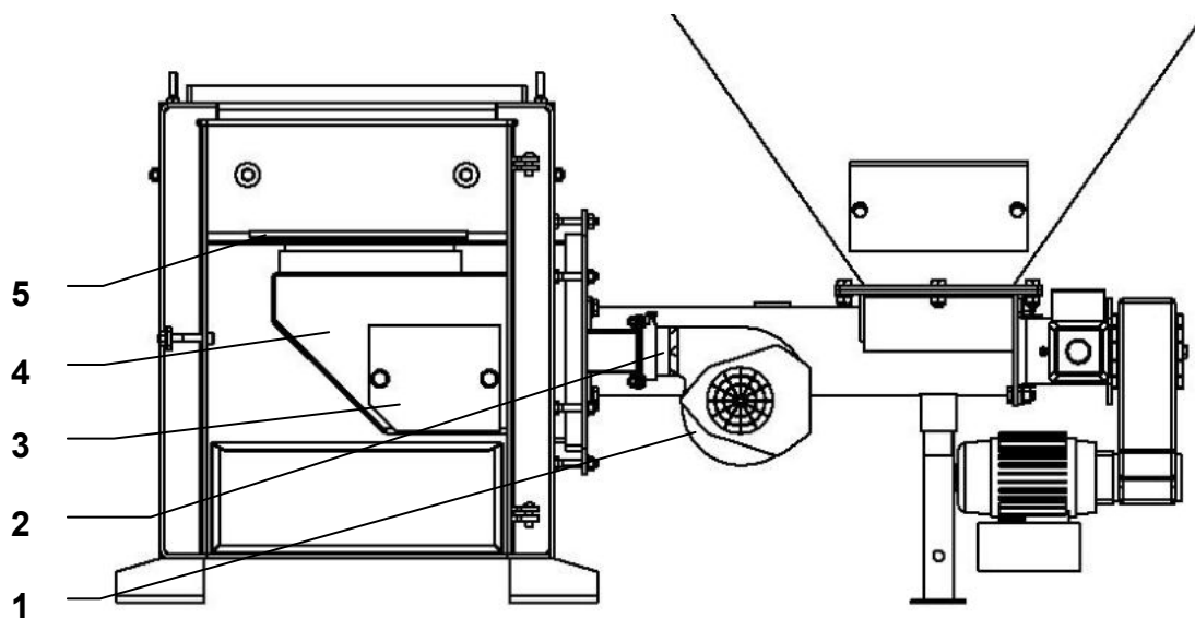
Obr. č. 7 Spalovací komora setu
