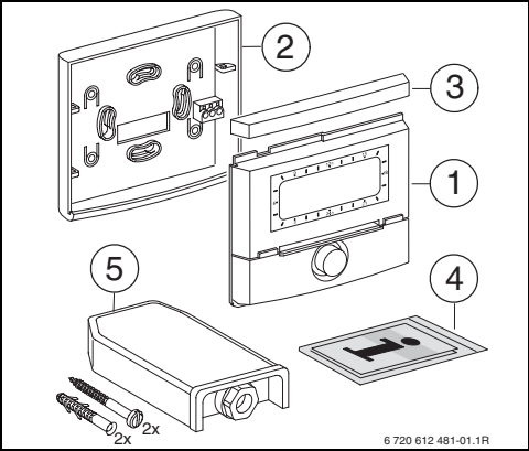
Obr. 2 Rozsah dodávky
