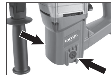
A szénkefe tartó helye az Extol Craft 401232 fúrókalapácsban 13. ábra
