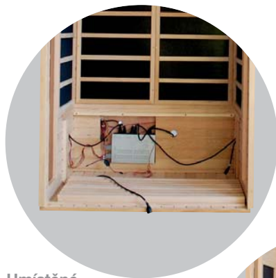
Umístěné podlahové topidlo
