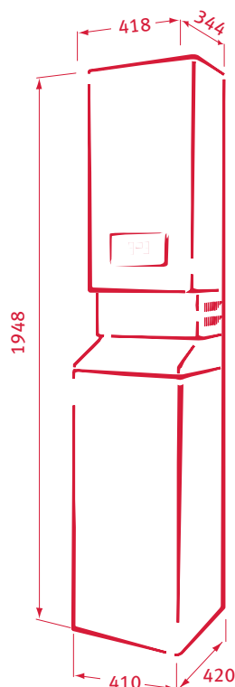
Sestava kotle Panther Condens 12 / 25 KKO se zásobníkem B60Z umístěným pod kotlem
