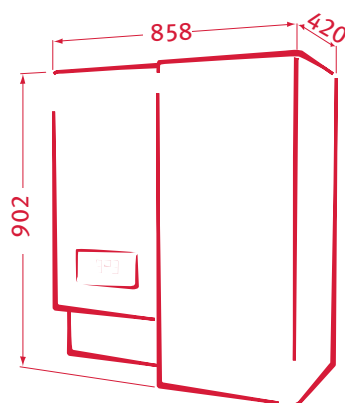
Sestava kotle Panther Condens 12 / 25 KKO se zásobníkem B60Z umístěným vpravo
