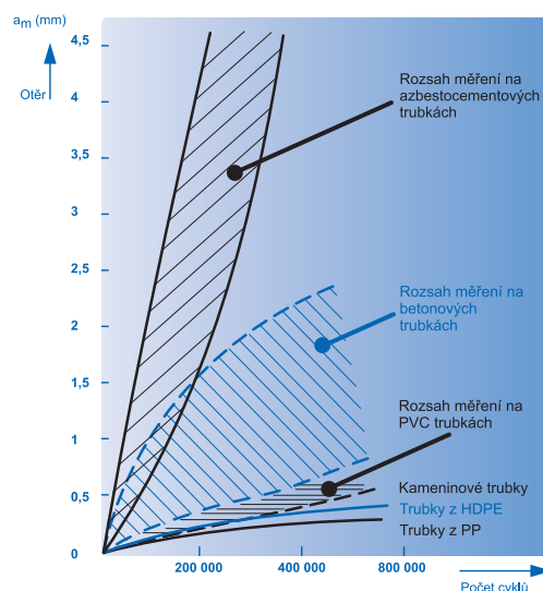
Odolnost trubek proti abrazi dle ČSN EN 295-3
