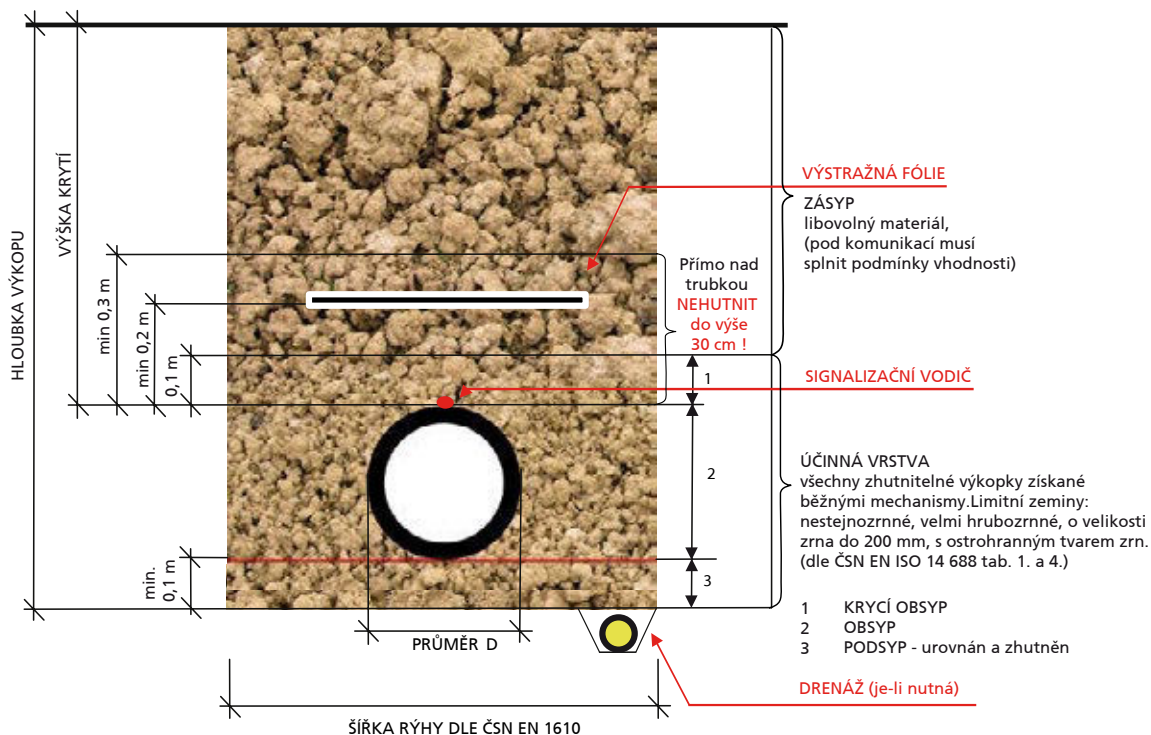
SCHÉMA ULOŽENÍ VODOVODNÍHO POTRUBÍ SUPERPIPE VE VÝKOPU
