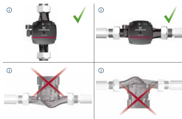
Rys. 7 Umiejscowienie skrzynki sterowniczej ALPHA SOLAR
