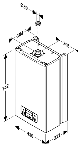
Gepard 23 MTV
