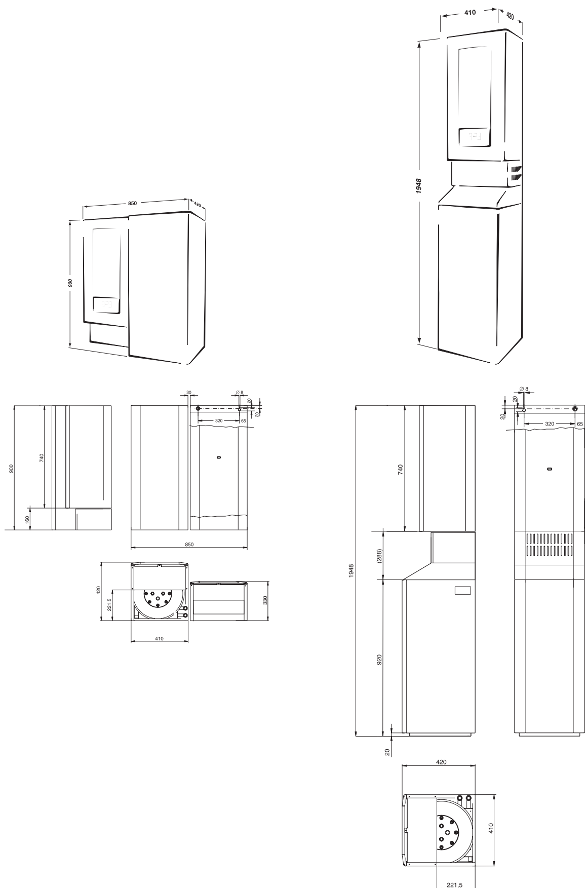
Boční sestava se zásobníkem B 60 Z (B)
