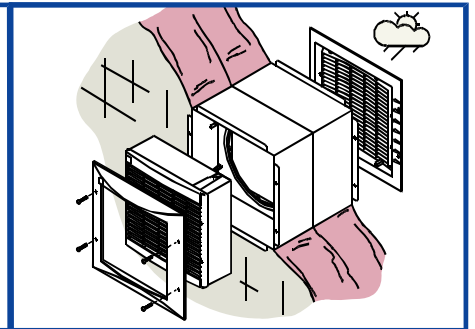
MONTÁŽ DO ZDI U VARIANTY RAB
