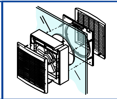
MONTÁŽ DO OKNA
