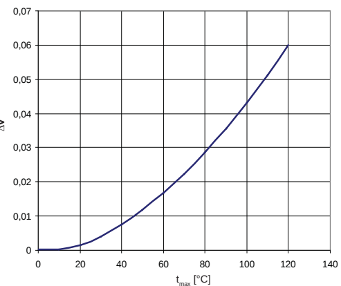
Graf závislosti poměrného zvětšení objemu vody Δv na t max
