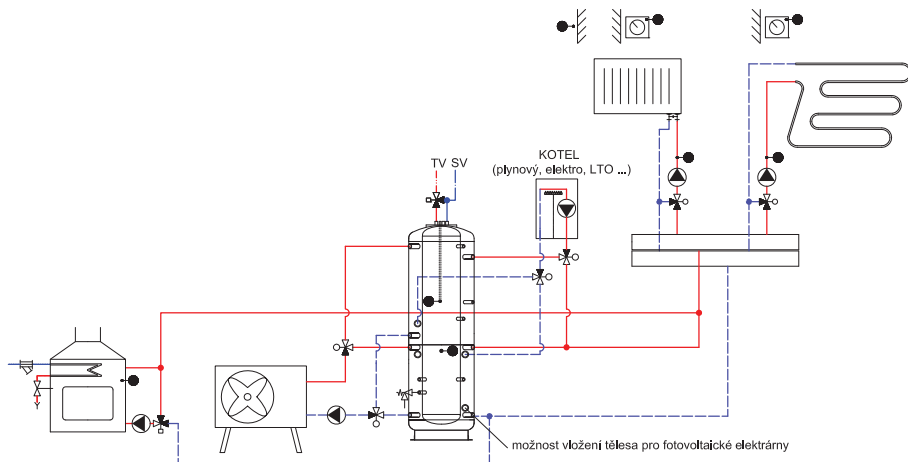
Schéma 2: Krb v kombinaci s tepelným čerpadlem a spínaným kotlem (na plyn, elektro, na LTO, ...)
