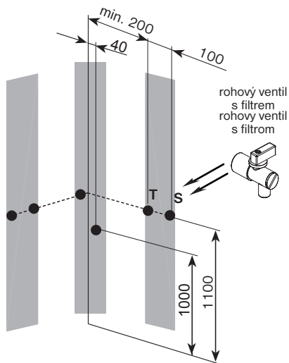
instalace na stěnu / rohu inštalácia na stenu / rohu
