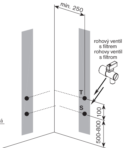
instalace na stěnu inštalácia na stenu
