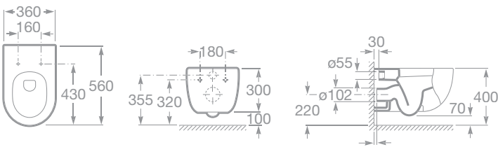
7346247000 Závěsný klozet, hluboké splachování 78012A0004 Klozetové sedátko s poklopem, s nerezovými úchyty 78012A2004 Klozetové sedátko s poklopem – Softclose, s nerezovými úchyty
