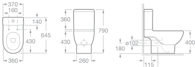
7342247000 WC mísa kombi, hluboké splachování, vario odpad, včetně instalační sady 7341240000 WC nádrž, armatura Dual flush – 3/6 nebo 3/4,5 l (nastavitelná) 78012A0004 Klozetové sedátko s poklopem, s nerezovými úchyty 78012A2004 Klozetové sedátko s poklopem – Softclose, s nerezovými úchyty
