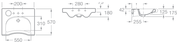
732724H000 Zdravotní umyvadlo 70 x 57 cm s instalační sadou 7506403207 Podomítkový sifon
