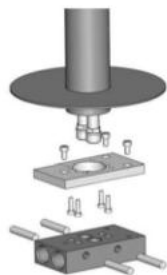
FISSAGGIO FIXING DEVICE
