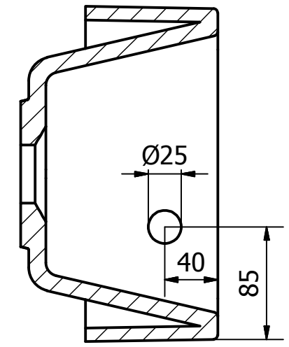
B-B ( 1 : 4 )
