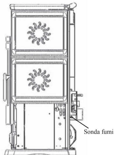
Vista laterale
