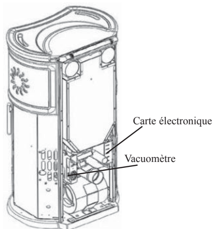
Vue latérale
