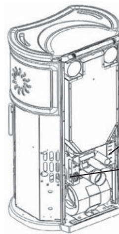
Seitenansicht
