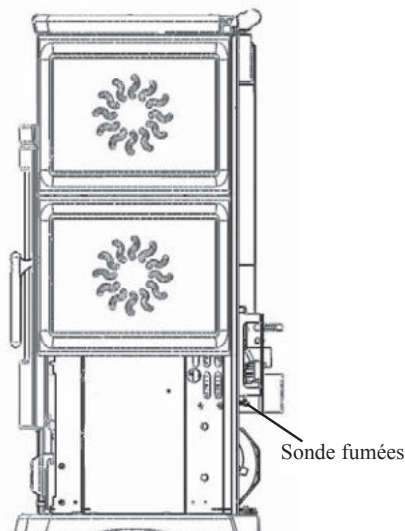
Vue latérale
