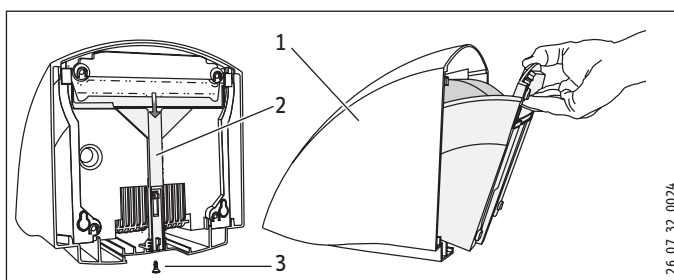
1 Cobertura da caixa
