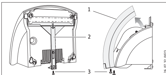
1 Cobertura da caixa
