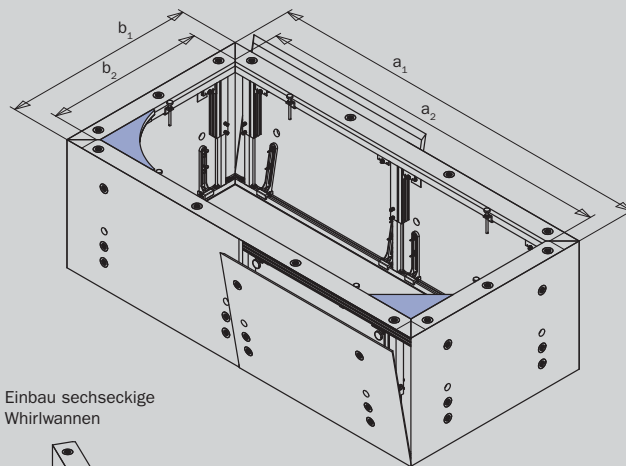
Einbau freistehende rechteckige, ovale und achteckige Whirlwannen
