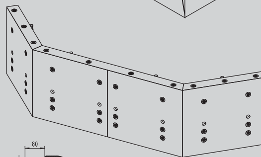
Einbau sechseckige Whirlwannen
