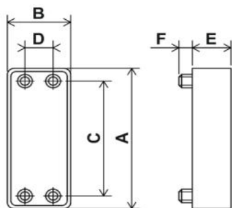
Rozměrové schéma
