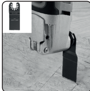
Obr.3, výřezy zanořovací pilový plátek
