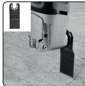
3. ábra. Besülyesztéses fűrészelés, fűrészlappal.
