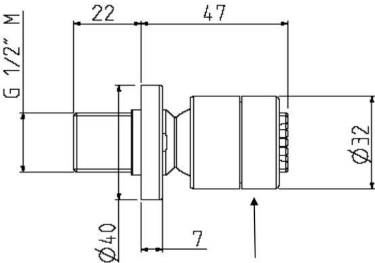
L'INCLINAZIONE DEL GETTO È REGOLABILE THE DIRECTION OF THE SPRAY IS ADJUSTABLE
